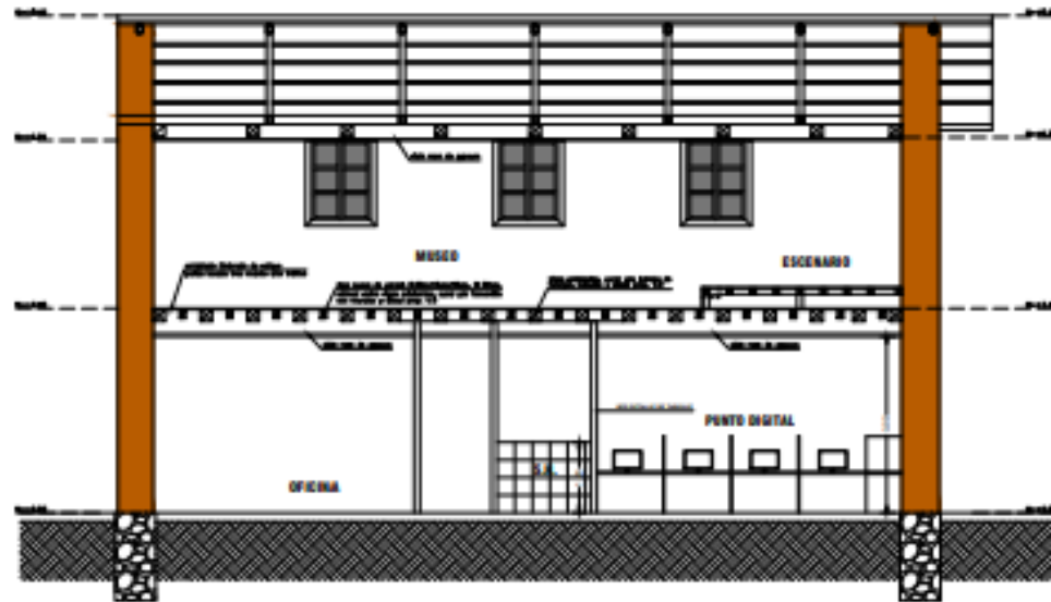
CORTE A-A ESCALA: 1:50 PROPUESTA
